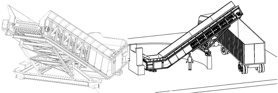
Gurtförderbänder in Modul-Bauweise, Optimiert für schnellste Montage Gurtbreite von 650 - 1200 mm
